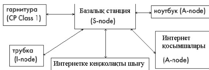
Сурет. HomeRF технологиясы бойынша құрылған желі құрылымы
